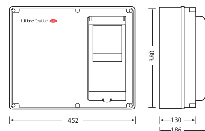
Ultra 3-fase verdampers module en Ultra 3-fase volledige module
